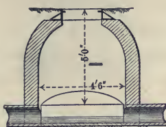
FIG. 2. SHALLOW MANHOLE.
